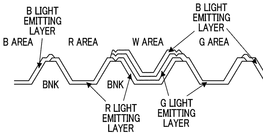
FIG.4E
